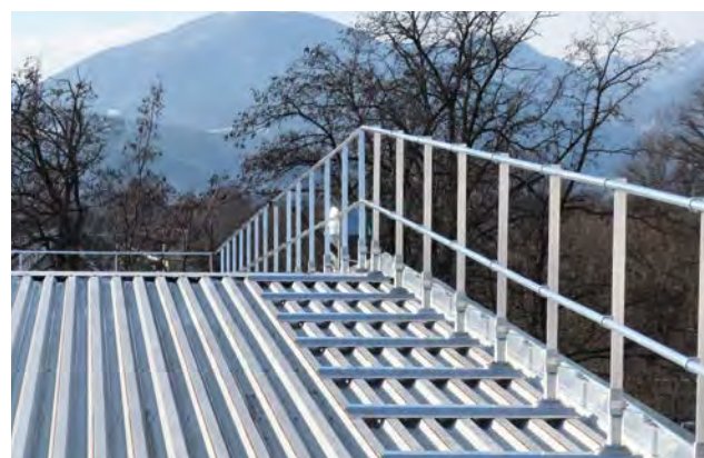
Sicherheitsgeländer Metalldach
