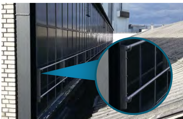
Sicherheitsgeländer Shed-Dach
